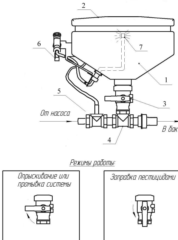
Рис. 4. Миксер.
