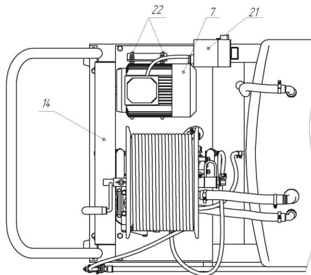
Рис. 1. Опрыскиватель ОТТ-400. Общий вид
